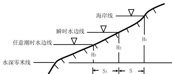
图H. 1 任意潮位线修正量计算参量示意图
